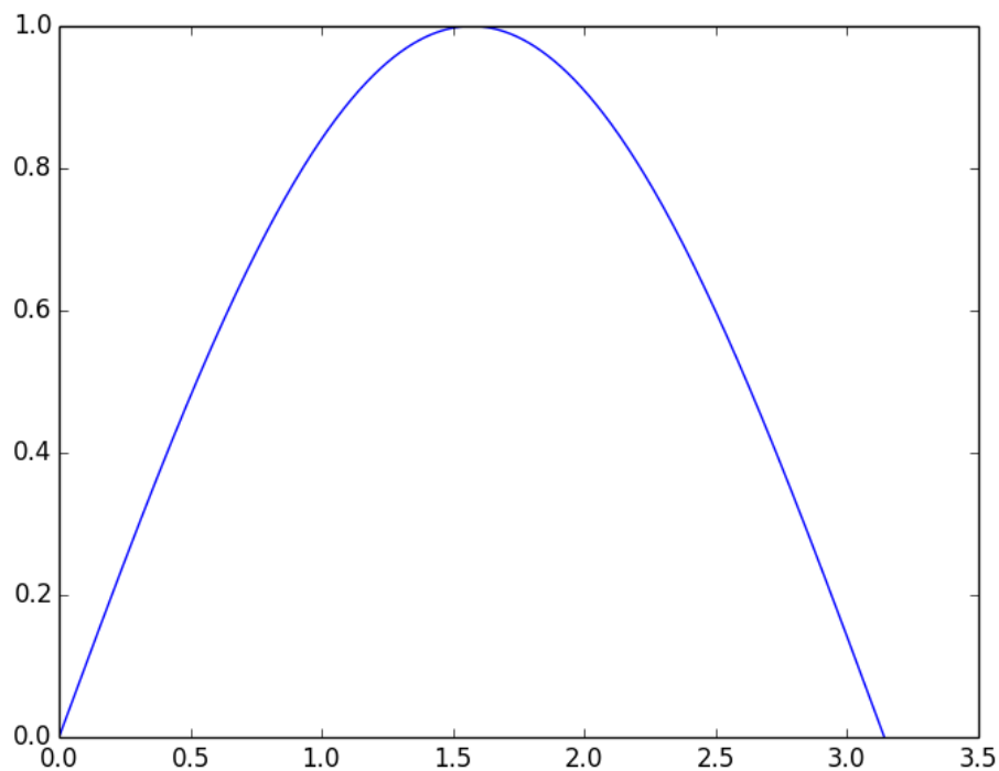
Abbildung 2: Sinus-Schwingung.
